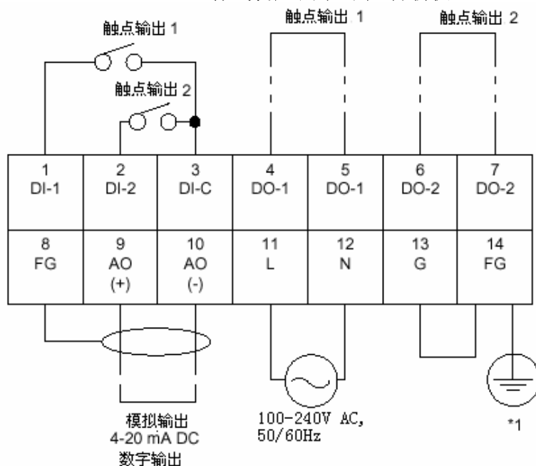
ZR202G 一体式氧化锆高温高湿分析仪
