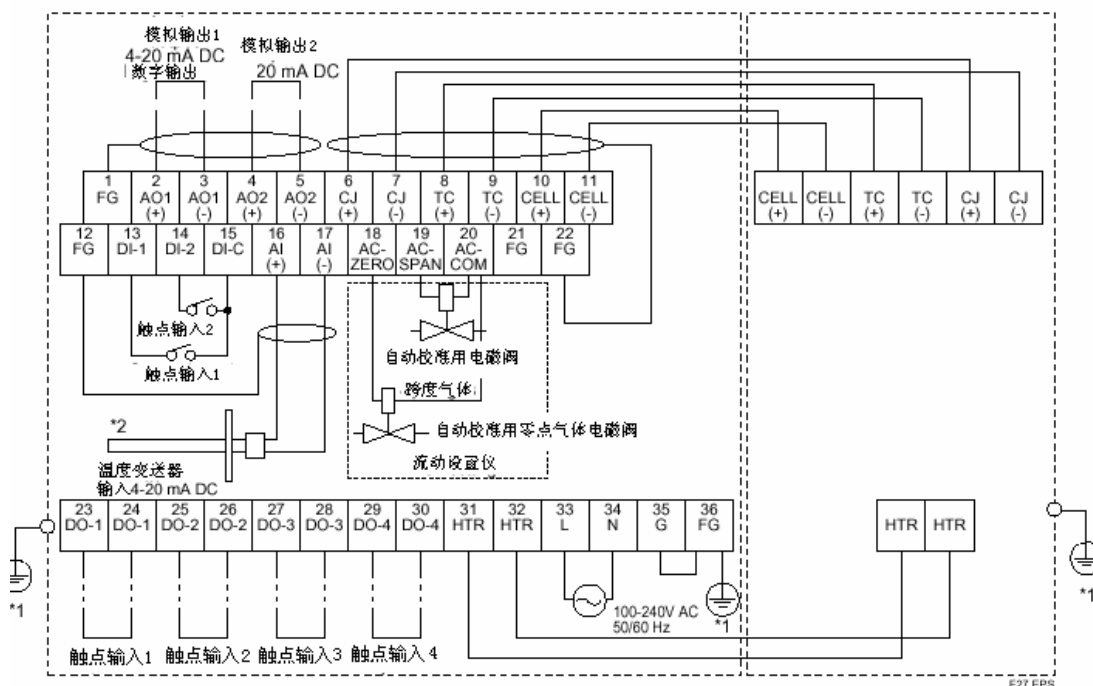
ZR22G 分离式氧化锆/高温湿度分析仪, 探头
